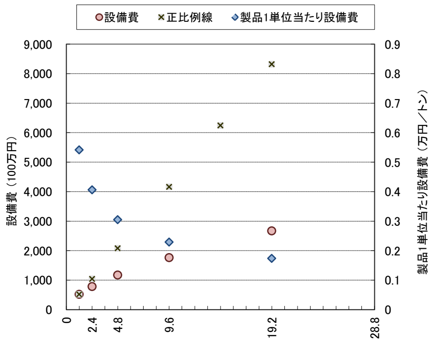
塩化ビニルモノマー工場の生産能力と設備投資額〔1965年〕
