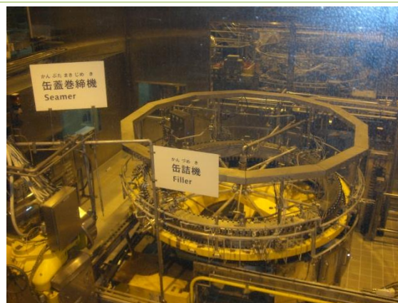
缶詰機と缶蓋巻締機：プルリング缶の蓋を毎分 150 缶の速さで締める。
